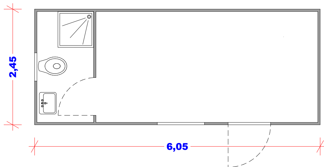
Monoblocco prefabbricato Tipo 1
